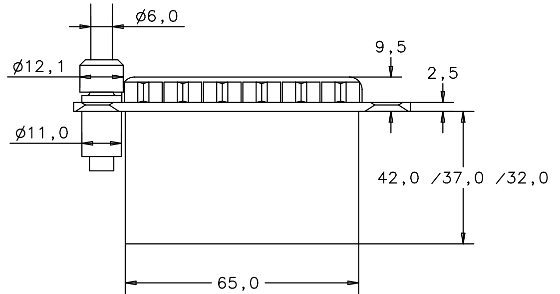
Rückansicht back view
