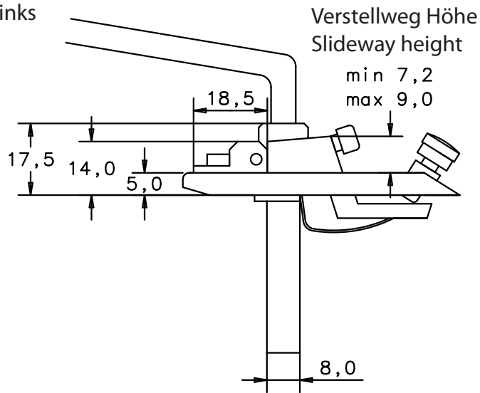
Seitenansicht von rechts side view right
