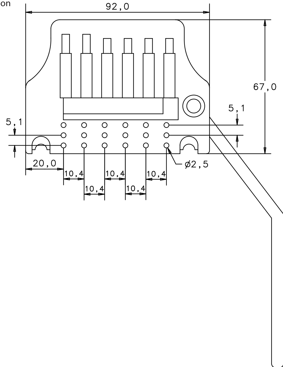
Untersicht bottom view
