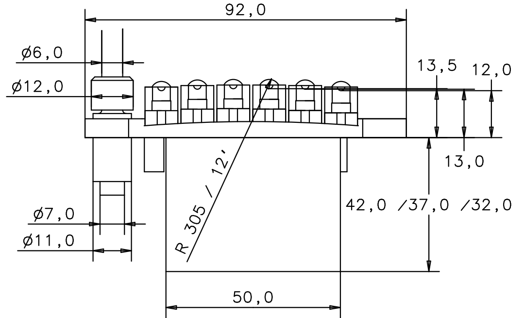
Rückansicht back view
