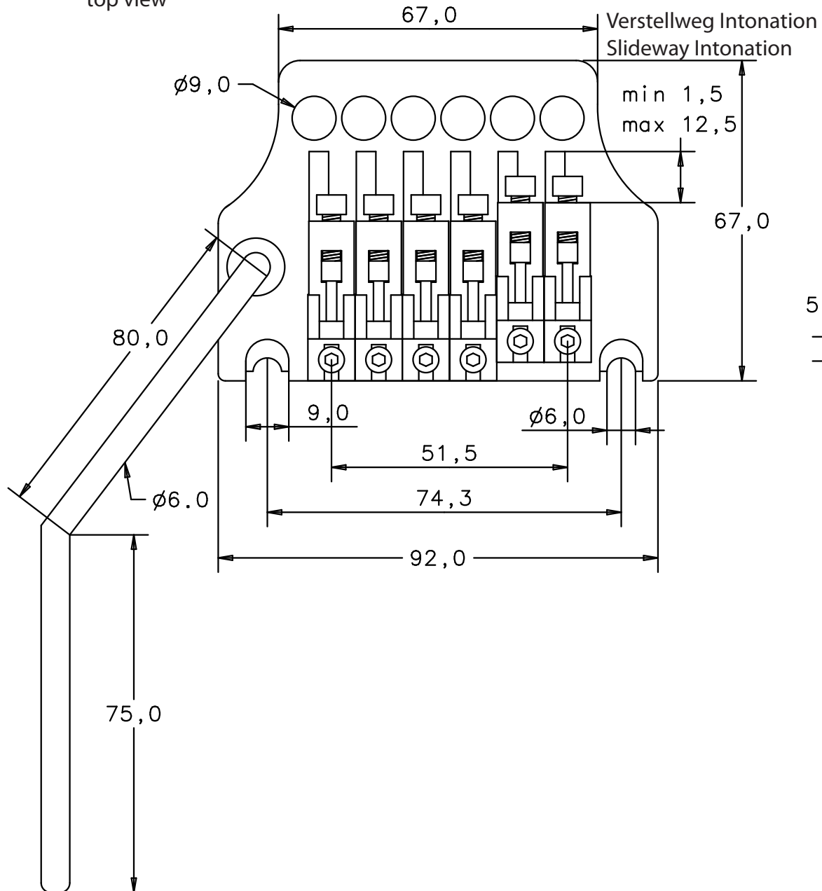
Draufsicht top view
