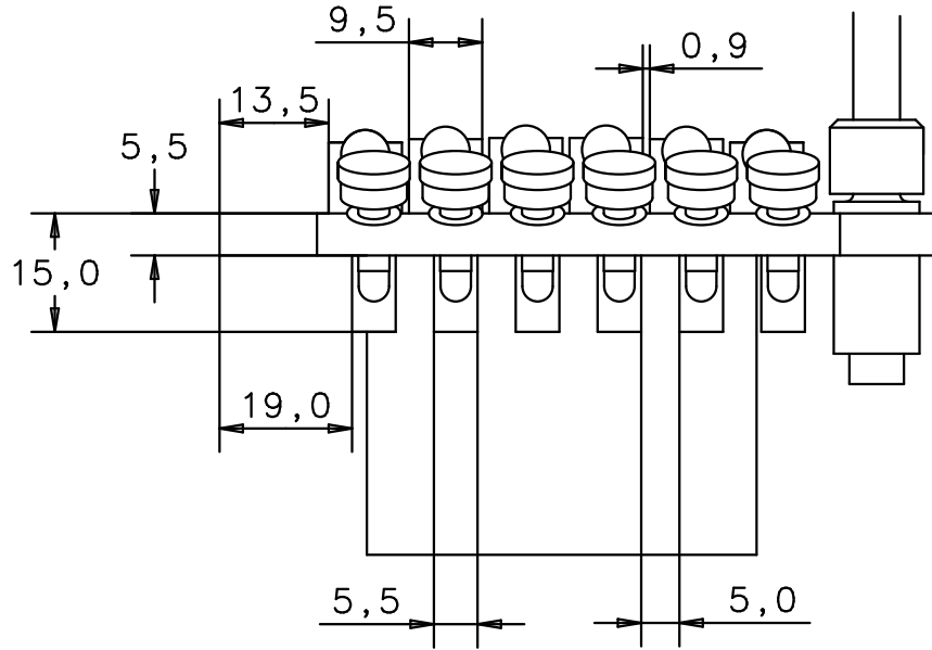
Seitenansicht von links side view left
