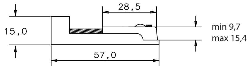
Seitenansichten side views
